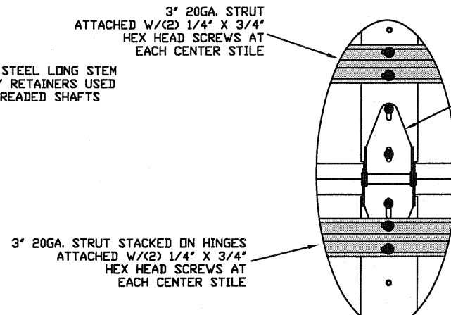
TYPICAL CENTER HINGE N.T.S.
