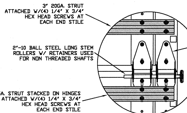
TYPICAL END HINGE N.T.S.
