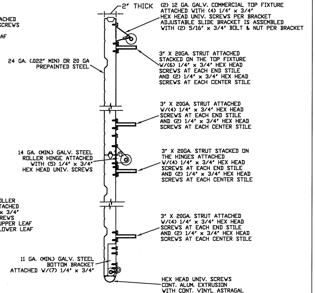
SECTION A-A (SIDE VIEW) N.T.S.
